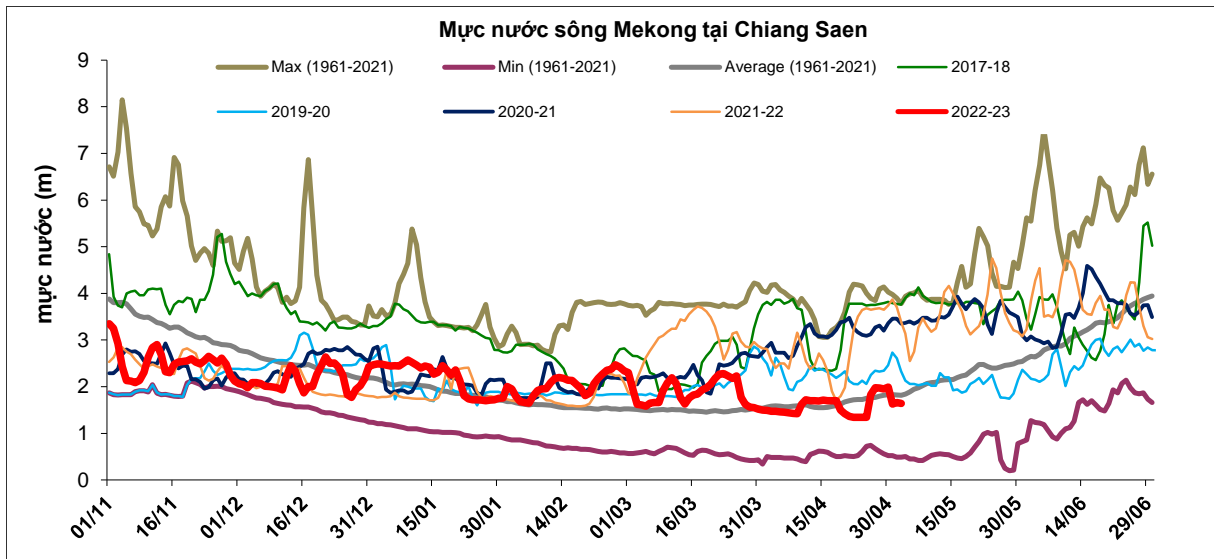
Hình 2. Diễn biến mực nước tại Chiang Saen –Thái Lan, cập nhật 03/5/2023
