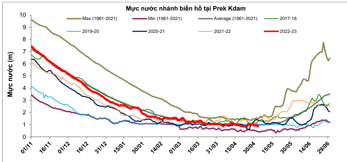
Hình 1. Diễn biến mực nước trạm Prek Kdam - Biển hồ, cập nhật ngày 03/5/2023
