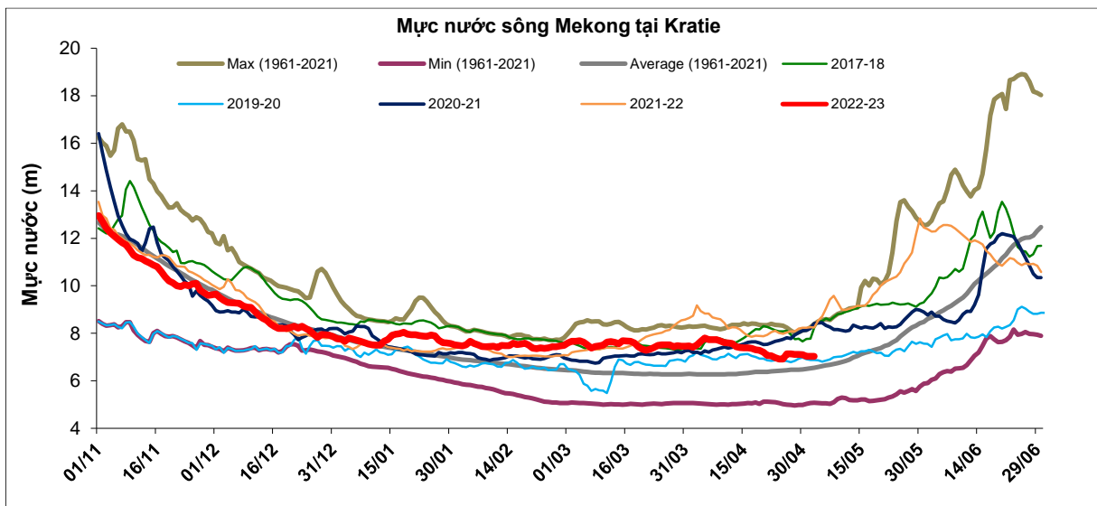
Hình 3. Diễn biến mực nước về qua trạm Kratie, cập nhật ngày 03/5/2023
